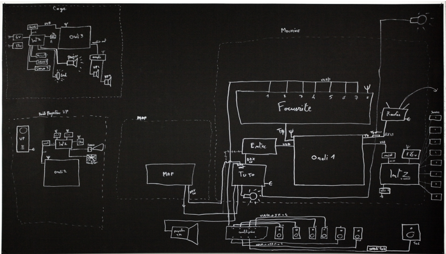
Schéma préparatoire de l'installation
